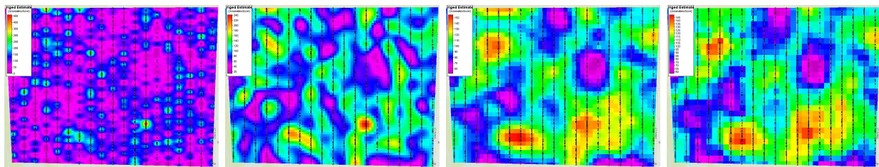
(a) 200 foot windows (b) 500 foot windows (c) 900 foot windows (d) 1,200 foot windows
