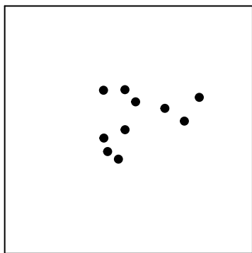
(d) Gaussian, max intensity 100
